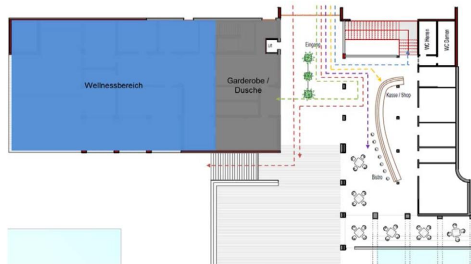
Grundriss Eingangsbereich / Besucherströme (Freibad, Hallenbad, Bistro, Post, Wellness)
